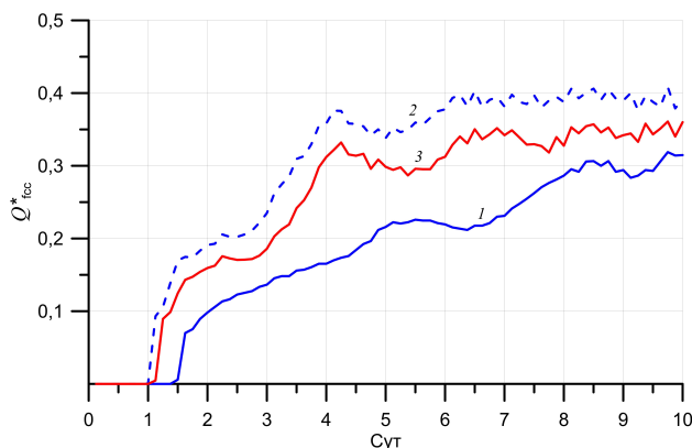
Р и с. 7. Расход пресной воды Q_{\text{fcc}}^* через разрез CD , по модельным данным, нормированный на пресноводный расход реки Q_{\text{fw}} = (S_a - S_0)/(S_a \cdot Q_r) , при S = 2 ЕПС и Q_r , равном 3000 \text{ м}^3/\text{с} (1), 8000 \text{ м}^3/\text{с} (2); при S = 6 ЕПС и Q_r = 8000 \text{ м}^3/\text{с} (3)
