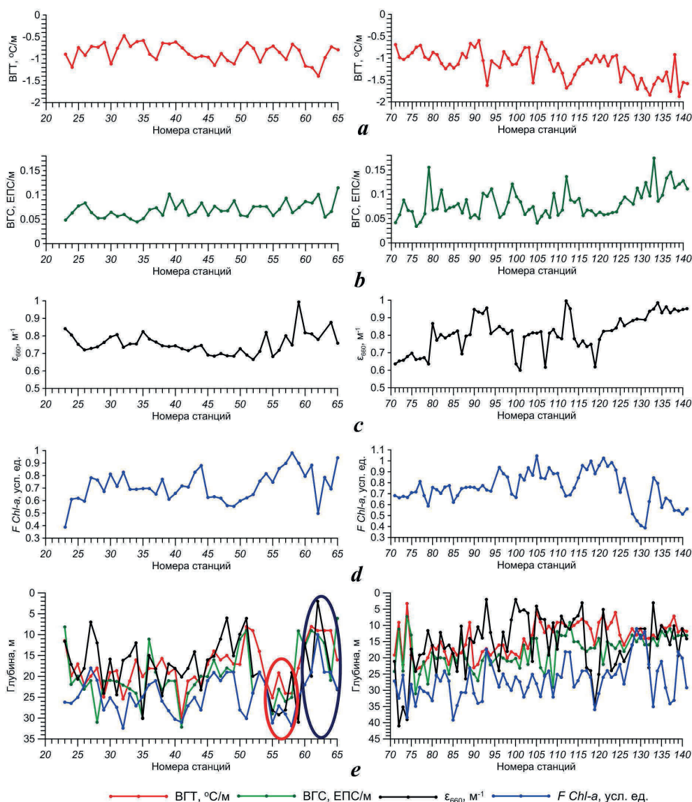
Рис. 8. Распределение значений основных максимумов ВГТ (а), ВГС (b), \epsilon_{660} (c), интенсивности F Chl-a (d) и глубин их залегания (e) на станциях, по данным 1-го (слева) и 2-го (справа) этапов 127-го рейса НИС «Профессор Водяницкий». Красным эллипсом выделены глубины залегания параметров на станциях в области Карадагского антициклона, синим – на станциях в области Феодосийского циклона
