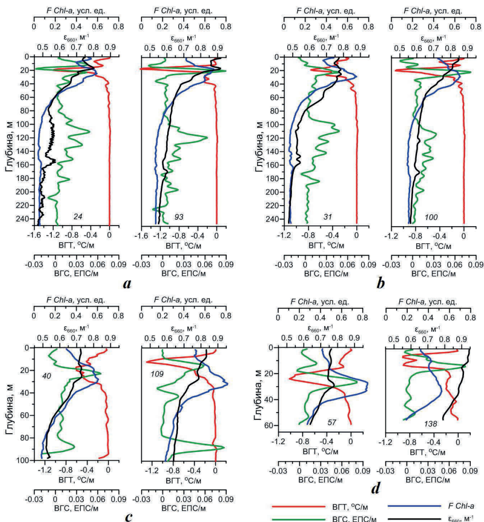
Р и с . 7 . Вертикальные распределения значений интенсивности F\ Chl-a , \epsilon_{660} , ВГТ и ВГС, зарегистрированных на станциях в тех же точках с интервалом в неделю в разных частях полигона. Номера станций указаны в нижней части графиков
