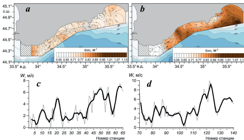
Р и с . 2 . Распределения значений \epsilon_{660} на поверхности ( a , b ) и скорости ветра W (м/с) ( c , d ) на станциях по данным 1-го ( a , c ) и 2-го ( b , d ) этапов 127-го рейса НИС «Профессор Водяницкий». Жирные кривые на фрагментах c , d – сглаживание скользящим средним по трем станциям
