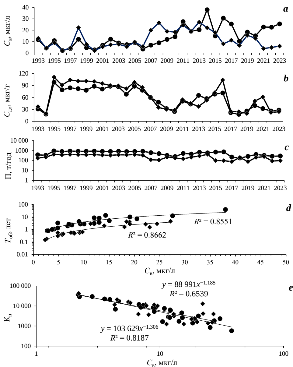
Р и с . 3 . Характеристики распределения цинка в открытой части моря (●) и Таганрогском заливе (◆): концентрация в воде (а); концентрация в поверхностном слое донных отложений (b); поток депонирования цинка в толщу донных осадков (c); период седиментационного оборота цинка в воде (d); зависимость изменения коэффициента накопления цинка донными отложениями от его концентрации в воде (e)
