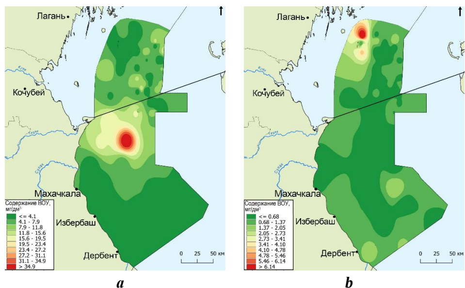
Рис. 3. Пространственное распределение взвешенного органического углерода ( \text{mg}/\text{dm}^3 ) в поверхностном слое воды весной 2020 г. (а) и осенью 2021 г. (б). Обозначение линии см. рис. 2
