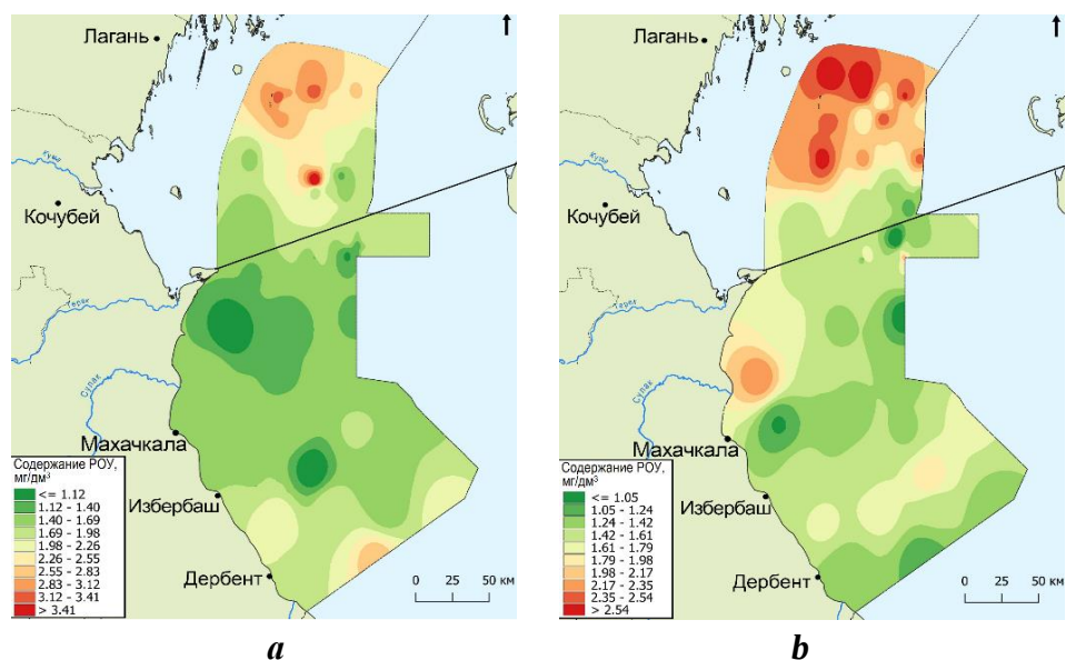
Рис. 2. Пространственное распределение растворенного органического углерода ( \text{mg}/\text{dm}^3 ) в поверхностном слое воды весной 2020 г. (а) и осенью 2021 г. (б). Линией обозначена граница между Северным и Средним Каспием
