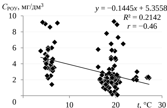
Р и с . 4 . Зависимость концентрации растворенного органического углерода C_{POY} ( \text{mg/dm}^3 ) от температуры воды ( ^{\circ}\text{C} ) в поверхностном слое в весенний период
