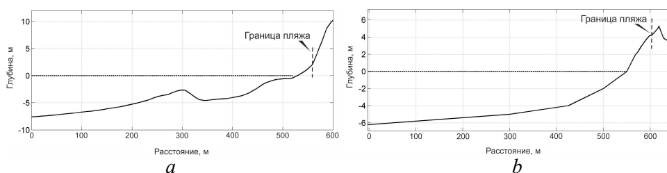
Р и с. 3. Береговые профили, характерные для участка Балтийской ( a ) и Октябрьской косы ( b ) F i g. 3. Coastal profiles typical for the regions of the Vistula ( a ) and Oktyabrskaya ( b ) spits
