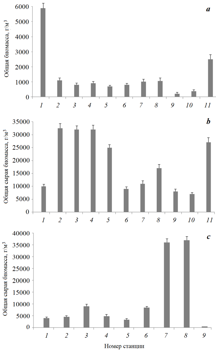
Р и с . 4 . Динамика распределения общей биомассы (а) и общей сырой биомассы (b, c) макрообрастания водозаборного туннеля ВТЭЦ-2 в разные годы: а, b – 2015 г.; c – 2001 г.
